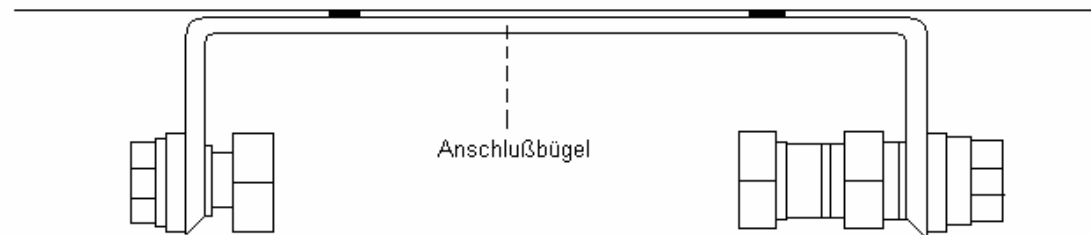
Wasserzählerbügel mit längenveränderlichem Ein- und Ausbaustück
