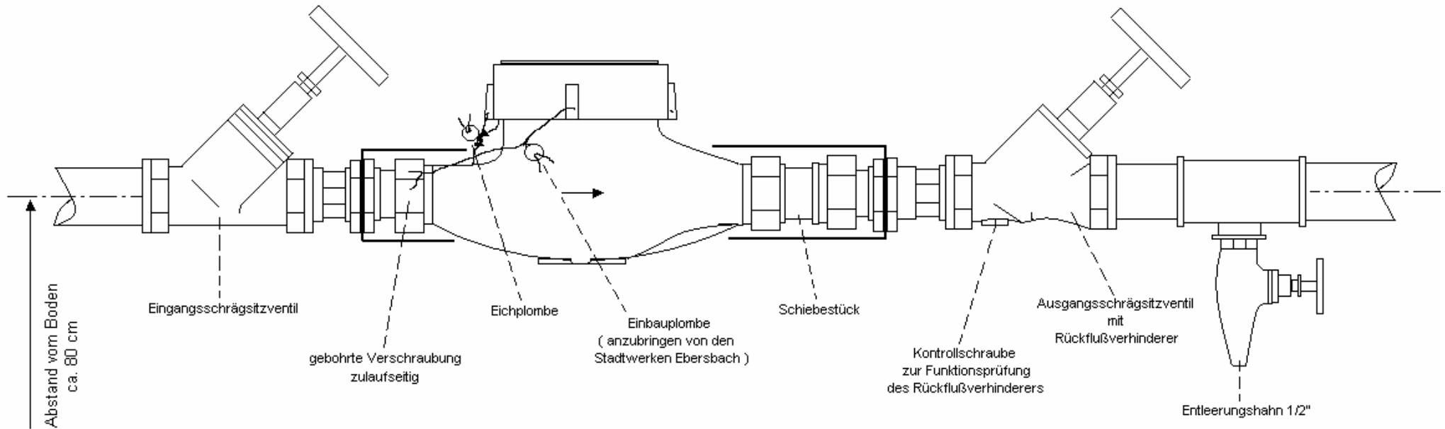
Wasserzähleranlage
